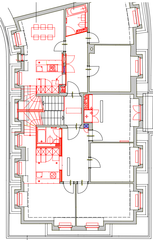
Grundriss Maisonettewohnung Dachgeschoss
