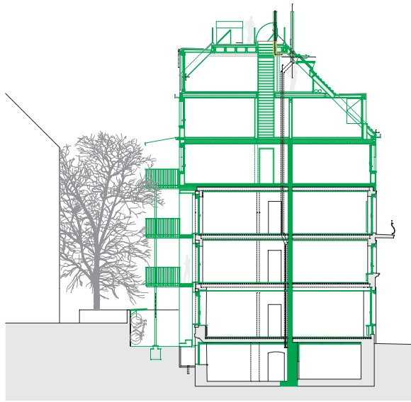
^ Querschnitt
