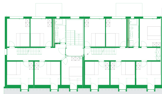
^ Grundriss 1. Dachgeschoss.
